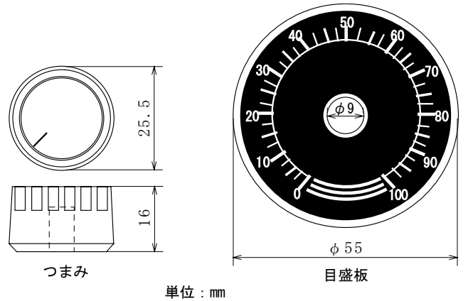
単位：mm
